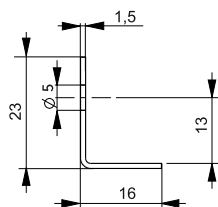
Przekrój A-A
